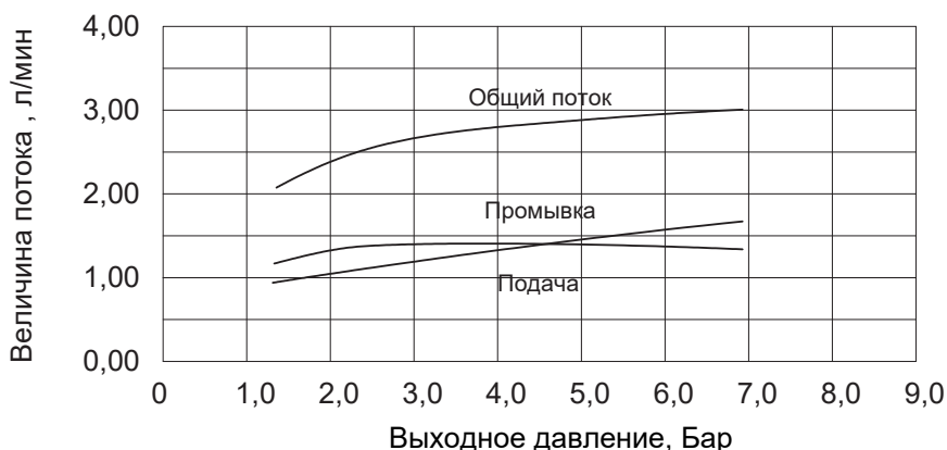
Инжектор 0 (Красный)
