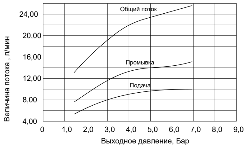
Инжектор 5С 1700/1710
