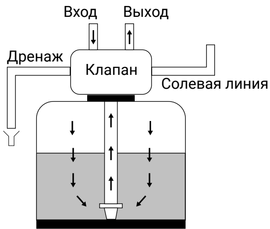
Рабочий режим
