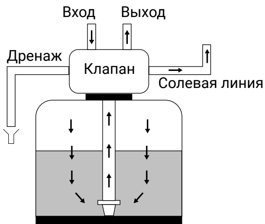
Заполнение бака-солерастворителя
